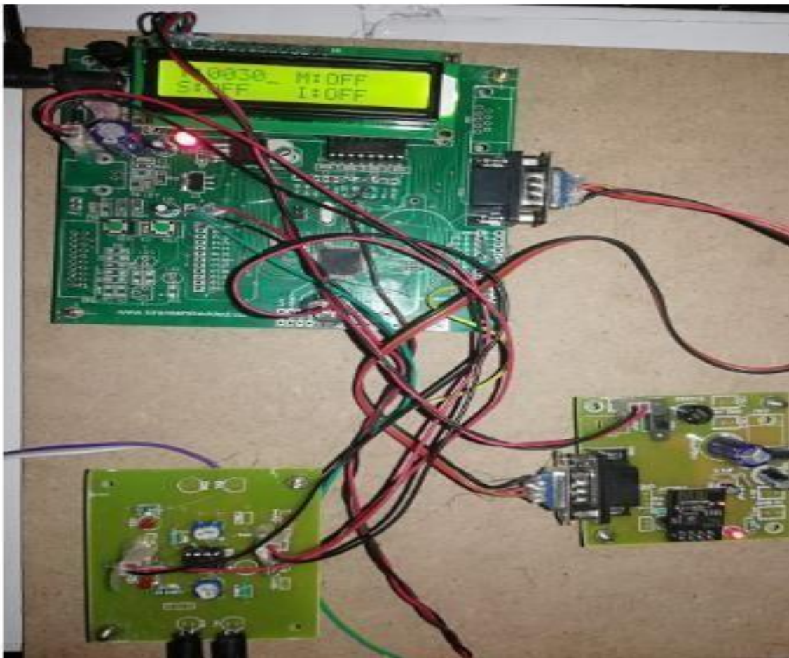
Fig.3.1.Hardwarekit.
